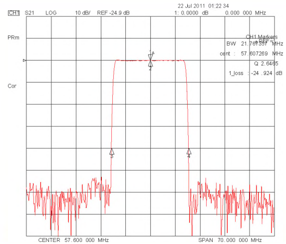
50dB Bandwidth
