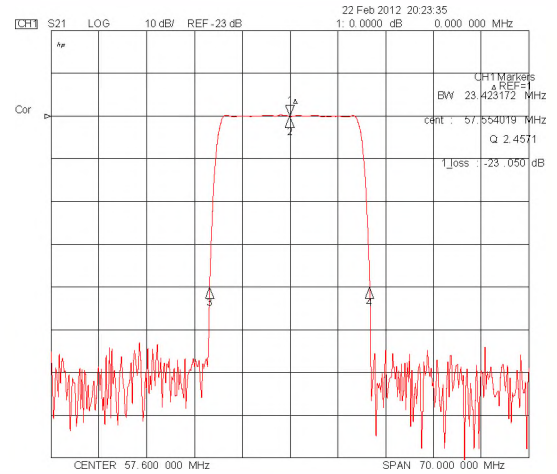
50dB Bandwidth
