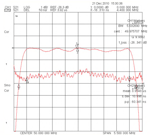
50dB Bandwidth
